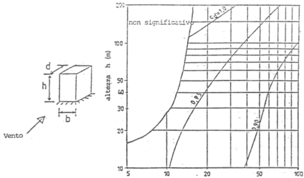
Fig. C.7.10 (a) - Edifici in c.a. o in muratura
