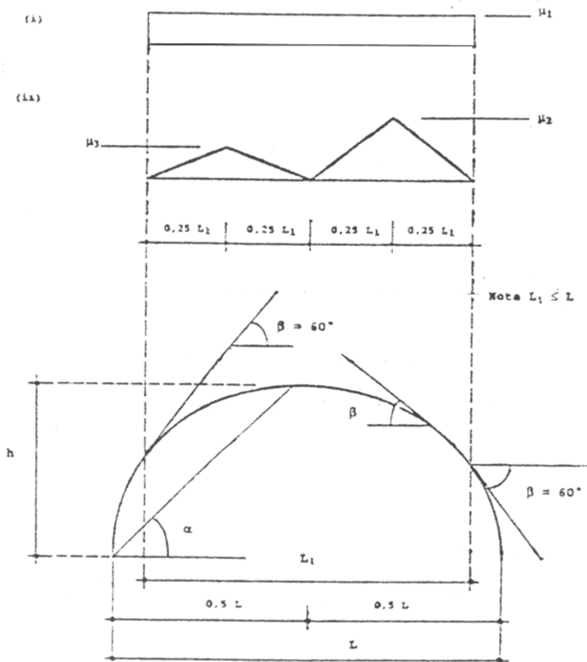
Fig. C.6.6 - Coefficienti di forma per coperture cilindriche.
