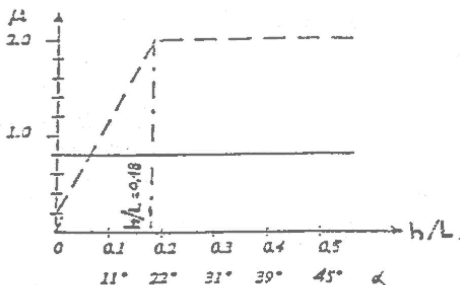
Fig. C.6.7 - Coefficienti di forma per differenti valori del rapporto freccia/luce.
