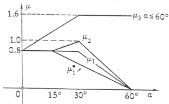
Fig. 6.2 - Coefficienti di forma per coperture a falde
