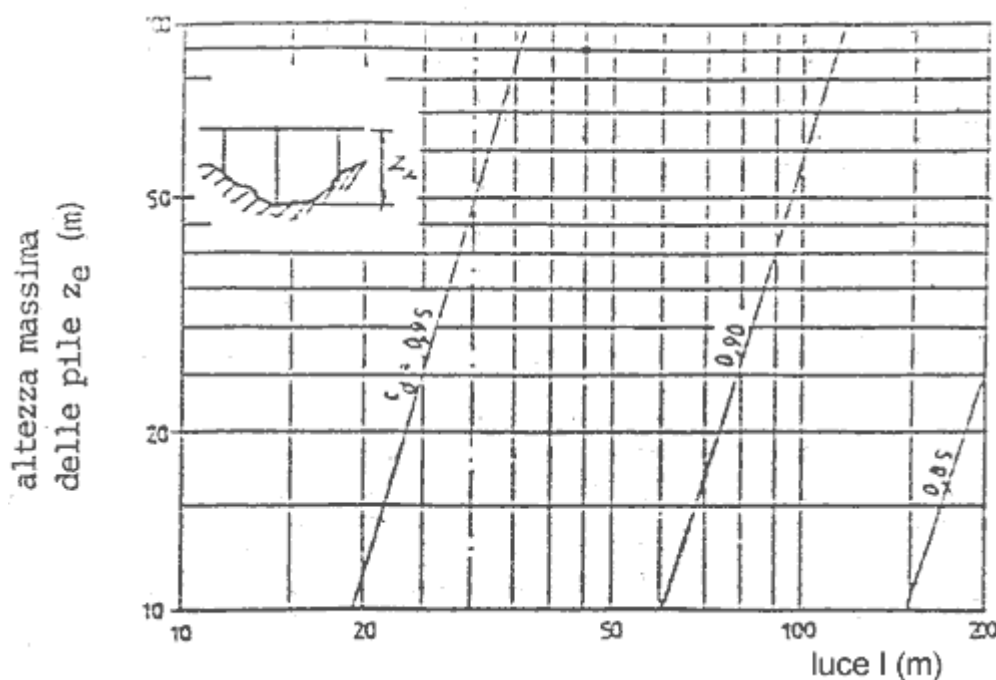
Fig. C.7.12 - Ponti stradali, ferroviari e pedonali
