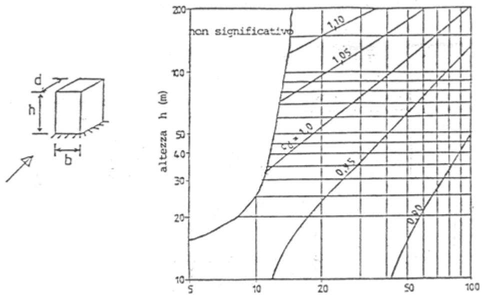
Fig. C.7.10 (b) - Edifici a struttura in acciaio
