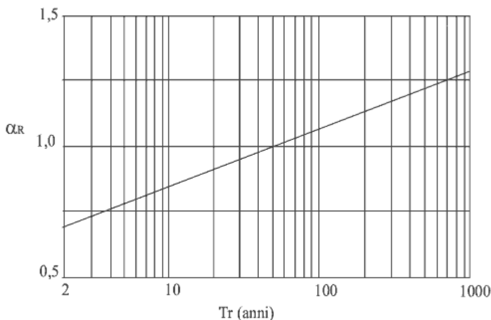
Fig. C.7.4 - Valori dell'azione del vento in funzione dell'intervallo di ritorno.
