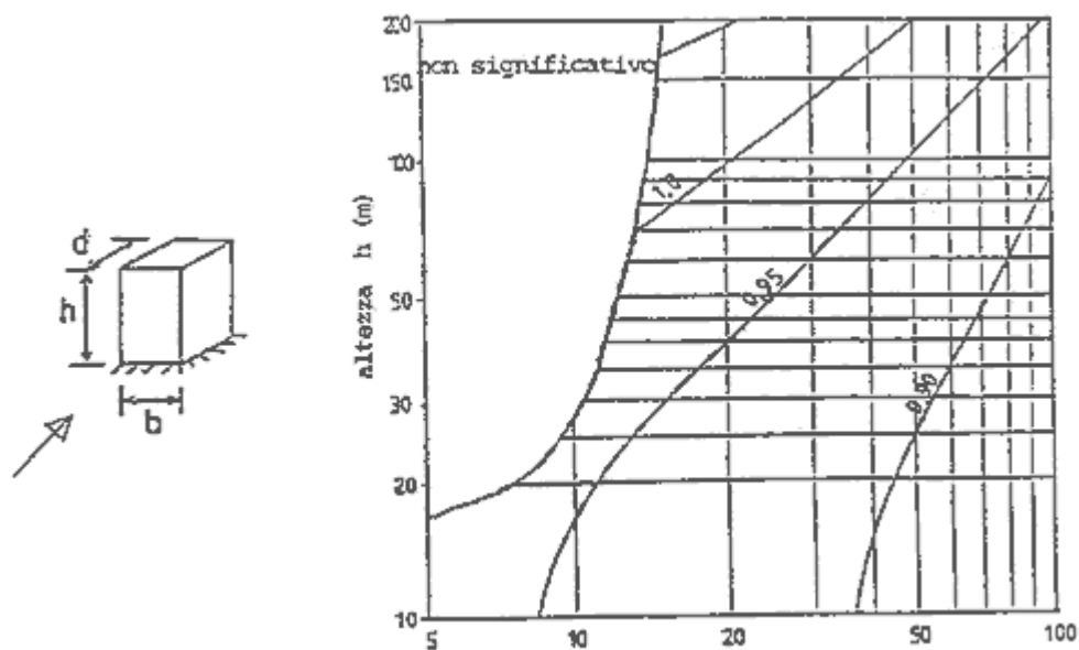
Fig. C.7.10 (c) - Edifici a struttura composta acciaio - calcestruzzo o edifici in acciaio con travi composte.
